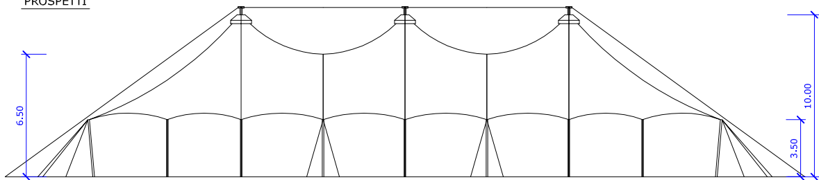
PROSPETTI
